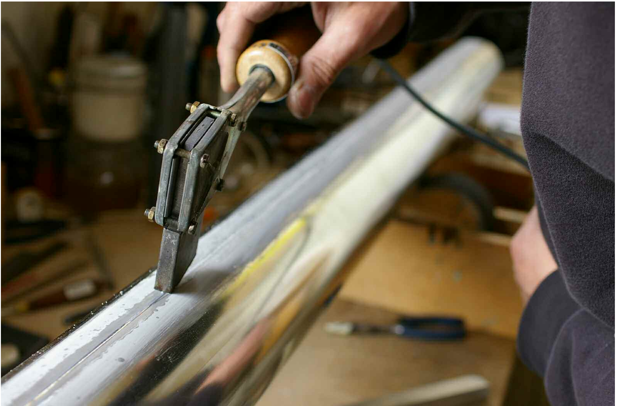
SOUDURE DU CORPS
