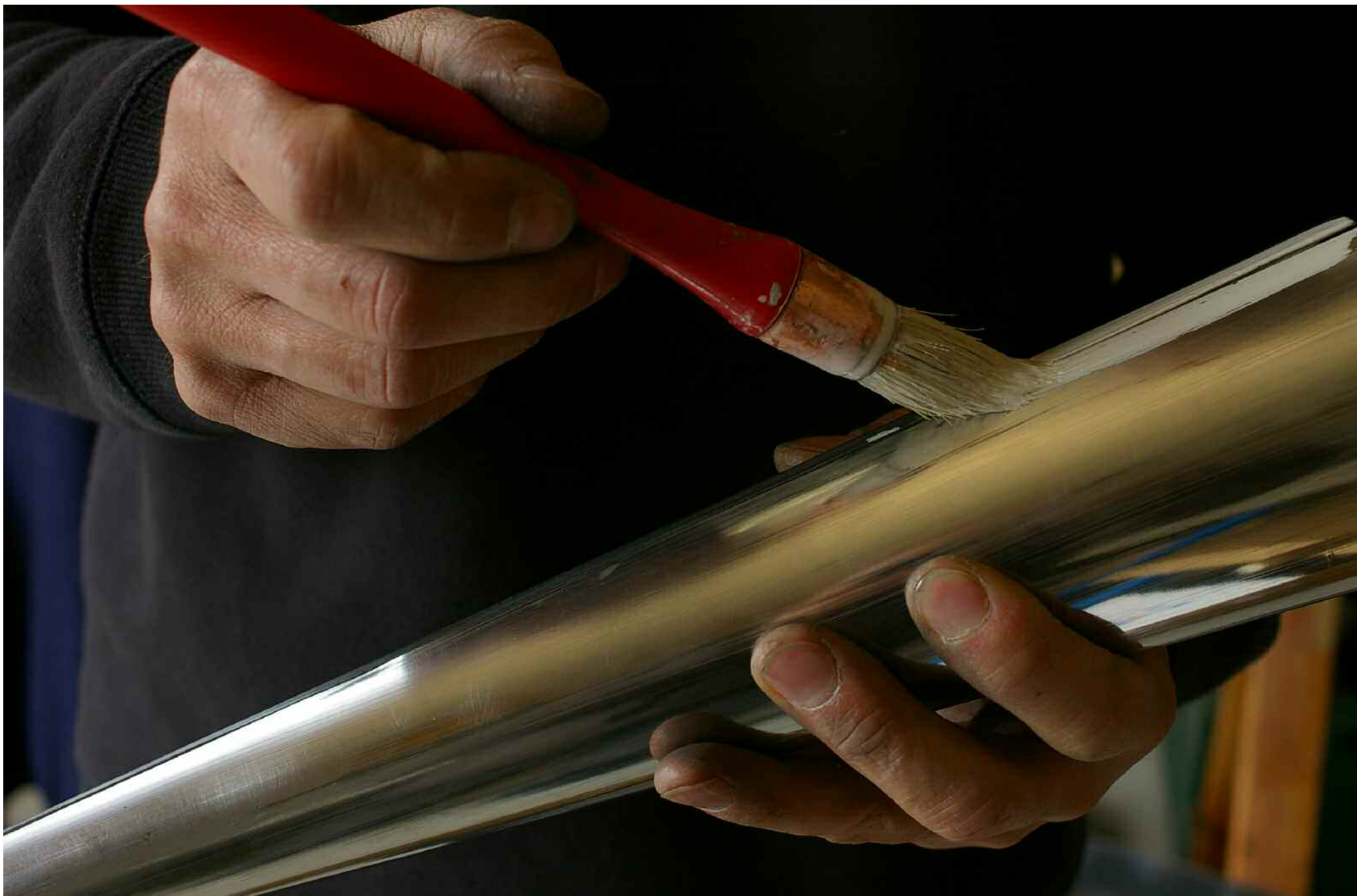
PEINTURE ISOLANTE POUR PRÉPARER À LA SOUDURE
